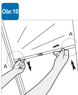
Obr.10 Unteres Gewicht in die Führungsleisten einfügen Detail Bild 11
