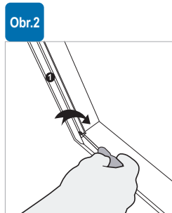
Obr.2 Schraube in untere Teil der Führungsschiene halbwegs ziehen
