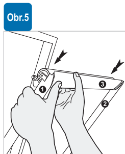
Obr.5 Stoffrollo in die Oberseite der Führungsleisten einsetzen (1+2)
