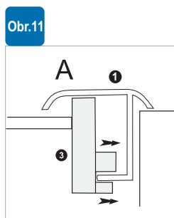
Obr.11 Mit unterem Gewicht zwischen Führungsleisten schräg bewegen (3). Linke Seite in die Führungsleiste 1+2) einführen. Wiederholen Sie diesen Vorgang mit der rechten Seite
